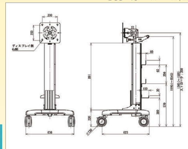
〈本体寸法図〉
